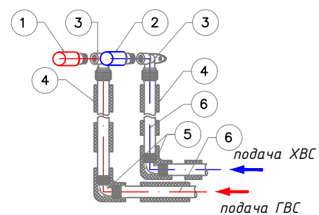
Подключение сантехприбора с холодной и горячей водой
